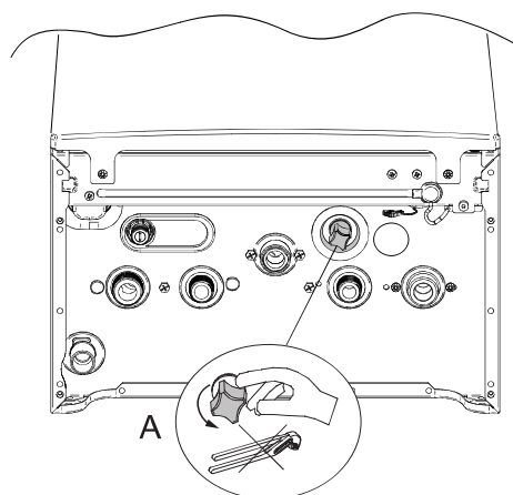
Fig.35 Umplerea instalației
