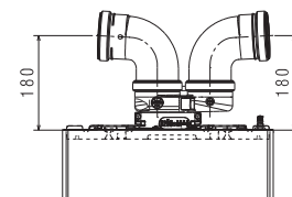
CONDUCTE DIVIZATE Ø80-80 mm CU ADAPTOR COMPACT
